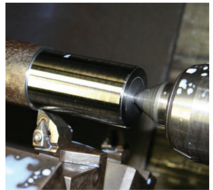
Obrábění čepu.
