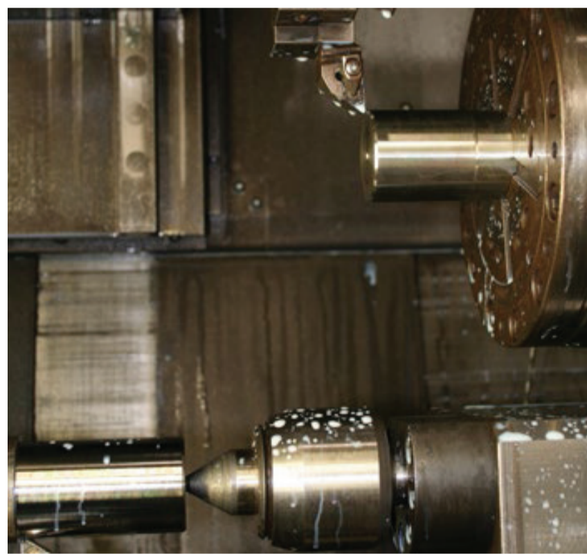
Zvýšení efektivity výroby díky současnému opracování dvou dílů.
